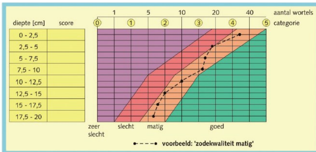
Meten doorworteling volgens de VTV methode (V&W 2007).
